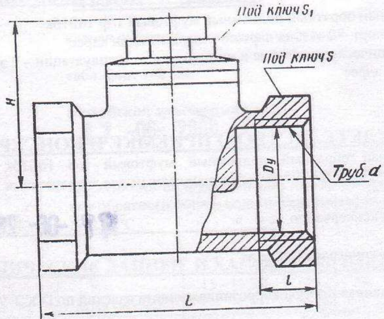
Рис. Клапан обратный подъемный муфтовый 16Б1бк
